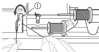
① Capac conducător de fir
